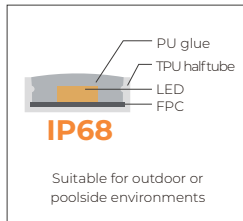
Filling PU
